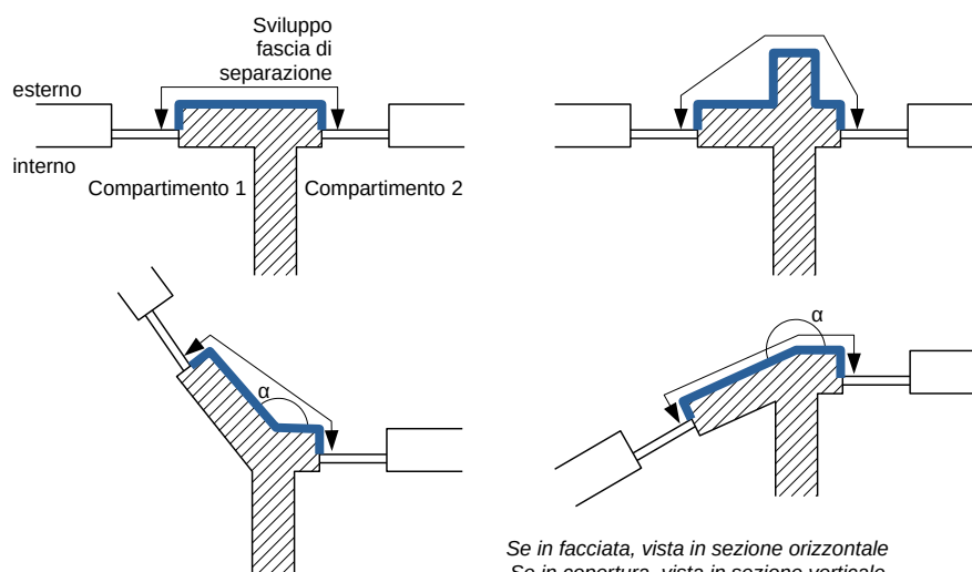
Illustrazione V.12-3: Esempi di fascia di separazione verticale in facciata o in copertura
