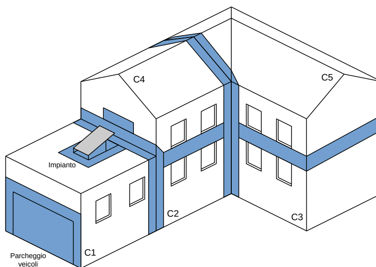
Illustrazione V.12-1: Esempio di fasce di separazione e protezioni per impianti e combustibili
