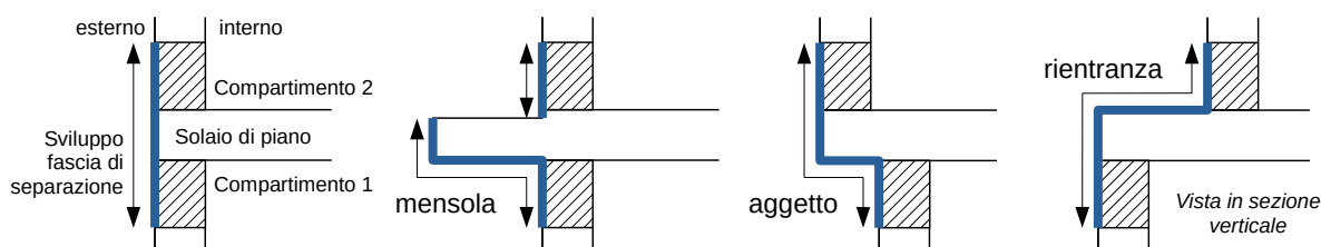
Illustrazione V.12-2: Esempi di fascia di separazione orizzontale in facciata
