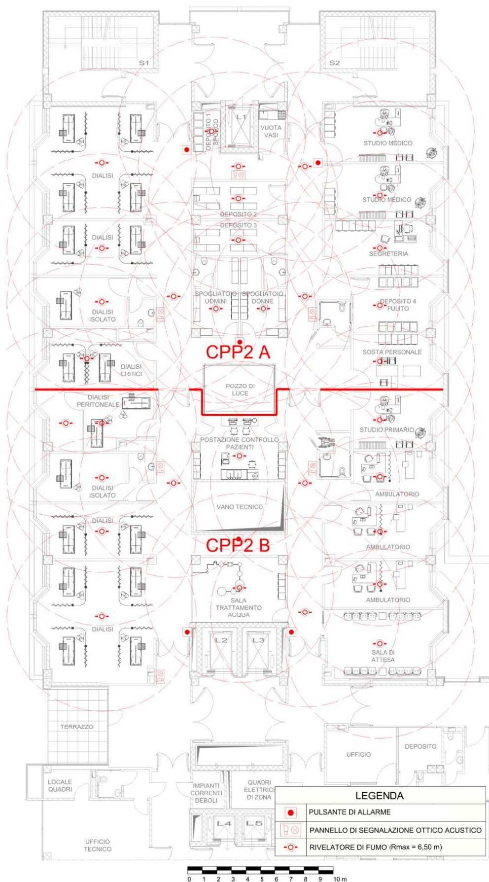
IRAI - Nuovo reparto Dialisi - Piano primo
